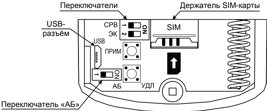
Рис.А2. Внешний вид платы прибора «GSM РОЗЕТКА ВЕКТОР» (видимая часть).
