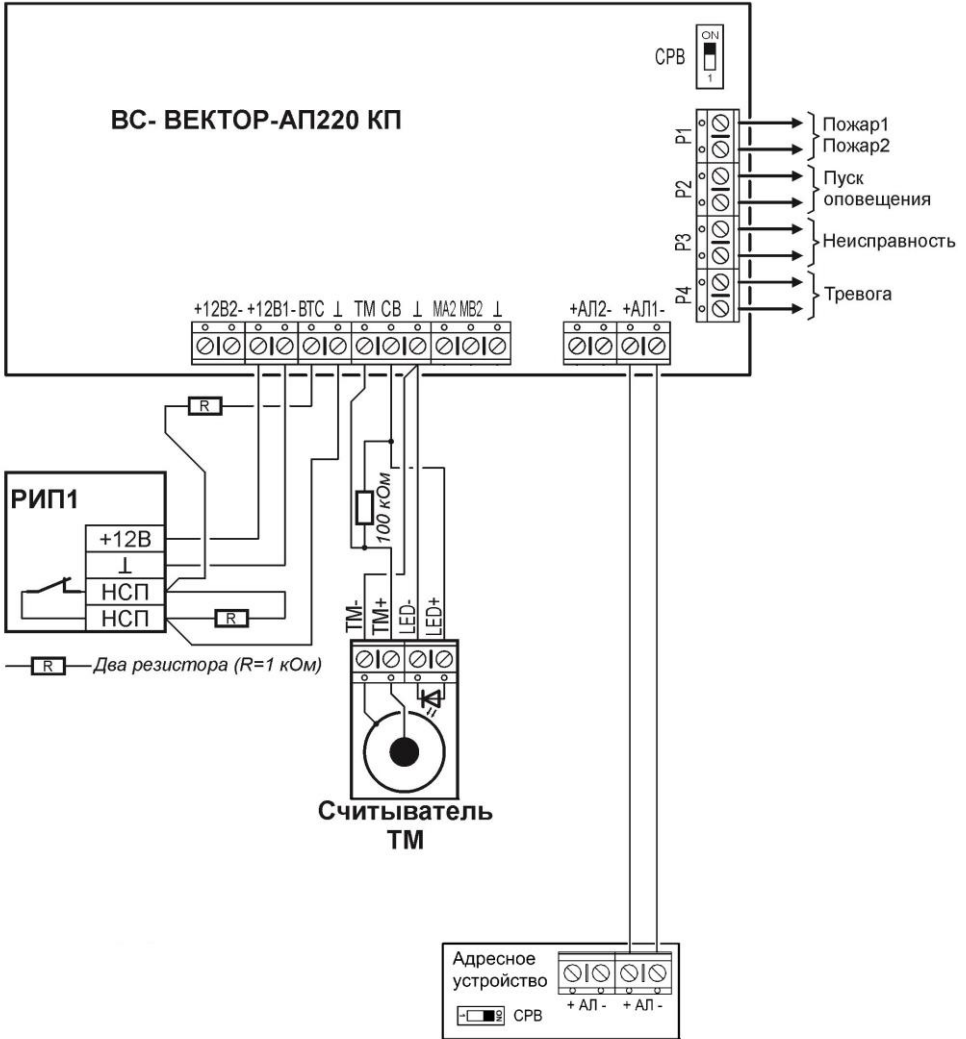
Рис.А1. Схема подключения к КП прибора считывателя ТМ и РИП. Схема подключения к КП прибора адресного устройства при креплении. Выходы реле
