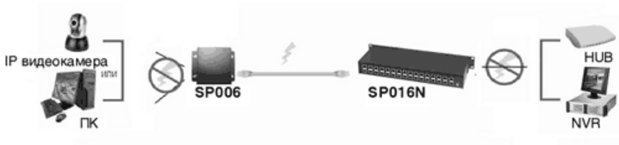
Рис.2 Подключение SP016N .
