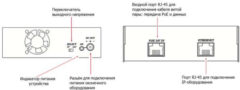
Рис.4 Разъёмы сплиттера IP06S.
