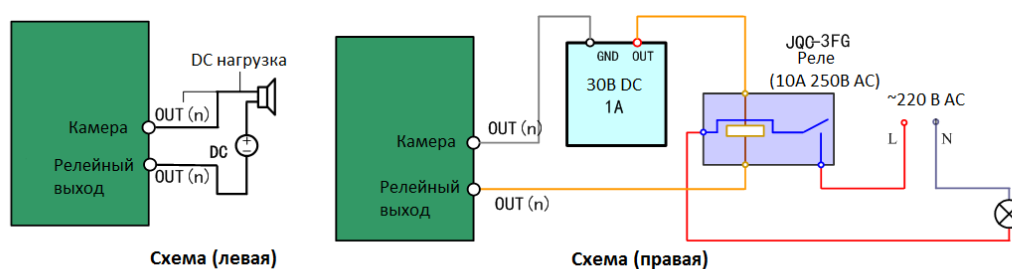
Рисунок А-11 Подключение тревожных выходов
