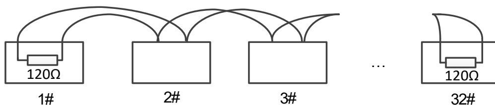
Рисунок А.6 Подключение RS-485 (1)
