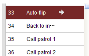
Рисунок 4-7 Специальные предустановки
