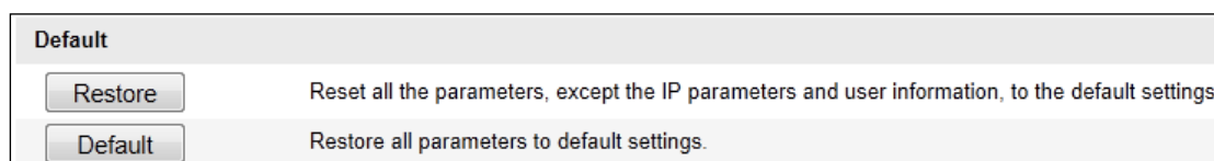
Рисунок 11-11 Восстановление настроек
