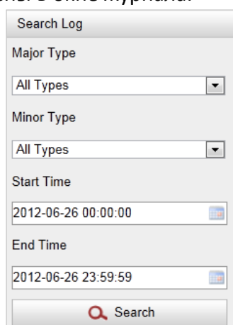
Рисунок 10-2 Поиск записей
