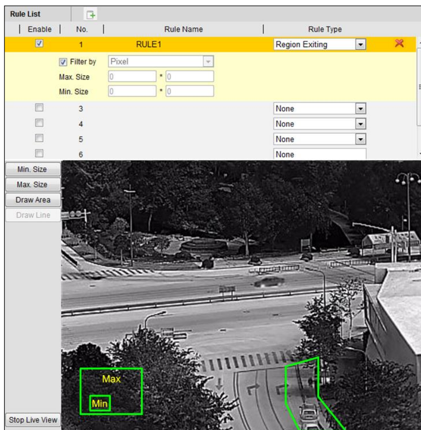
Рисунок 7-13 Рисование области
