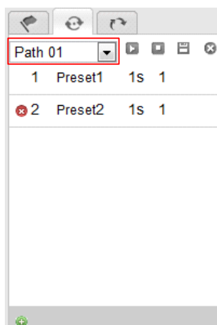
Рисунок 4-9 Вызов патруля
