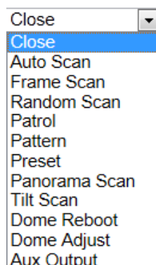
Рисунок 5-10 Типы задач
