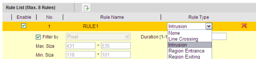
Рисунок 7-6 Список правил
