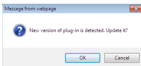
Рисунок 3-3 Установка плагина (1)
