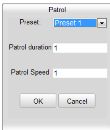
Рисунок 4-8 Добавление предустановок
