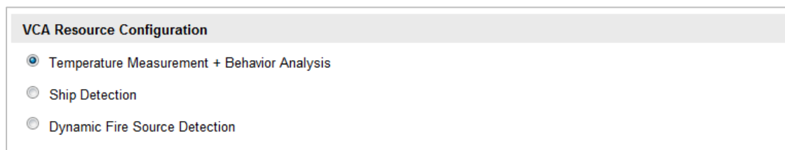
Рисунок 7-1 VCA информация
