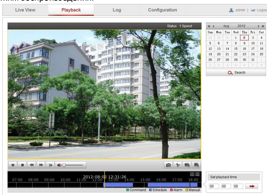
Рисунок 9-1 Меню воспроизведения
