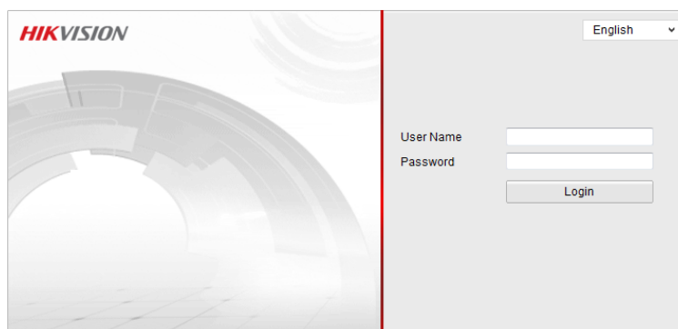
Рисунок 3-1 Меню авторизации
