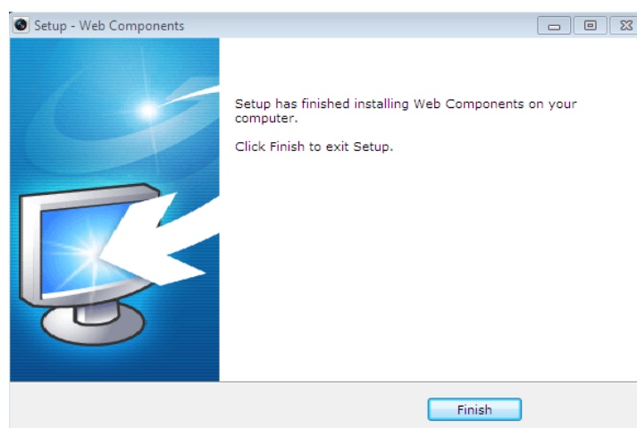
Рисунок 3-5 Установка плагина (3)
