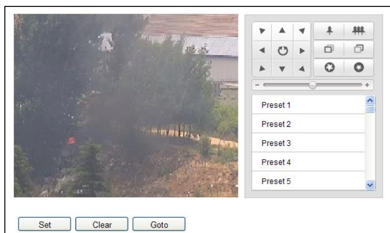
Рисунок 5-3 Настройка PTZ
