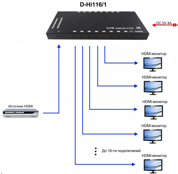
Рис.3 Типовая схема подключения HDMI-разветвителя D-Hi116/1
