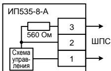
Рис.2 Схема подключения к ШПС ППКП «Гранит» «Кварц» «Карат»
