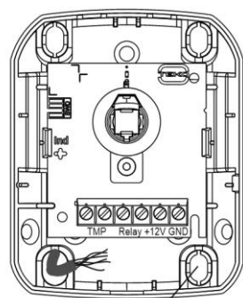
Заглушка отверстия для проводов
