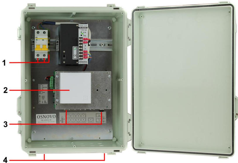
Рис.2 Коммутатор SW-60812/W, вид внутри
