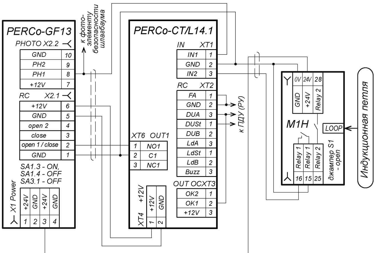
Рисунок 16. Вариант схемы подключения датчика индукционной петли для управления слягбаумом с односторонним проездом
