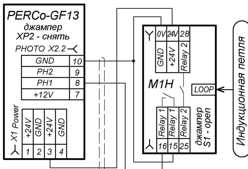
Рисунок 14. Схема подключения одноканального датчика M1H в качестве элемента безопасности и датчика проезда
