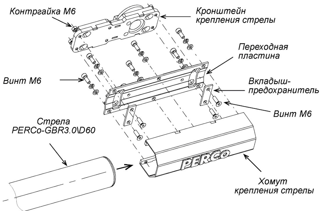
Рисунок 11. Монтаж стрелы PERCo-GBR3.0\D60
