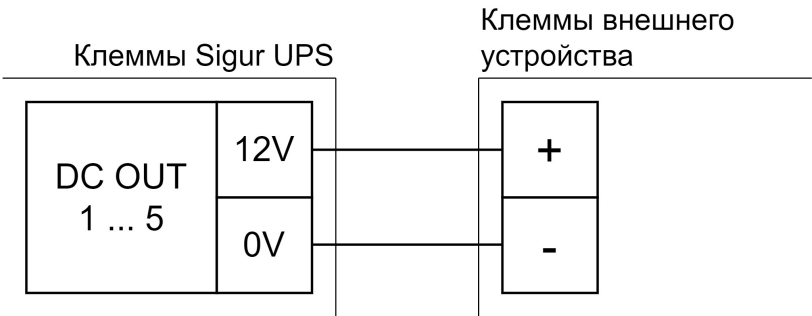
Схема подключения нагрузки к контактам выходных каналов.
