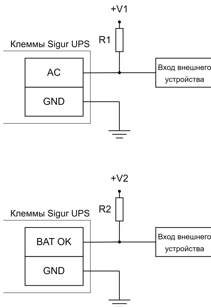
Схема подключения внешних устройств к выходам типа «Открытый коллектор».
