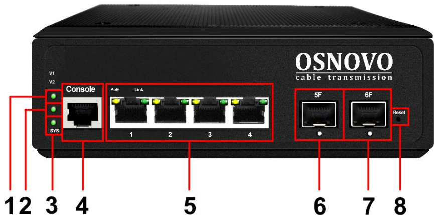
Рис.1 Коммутатор SW-80402/IL, разъемы, кнопки и индикаторы
