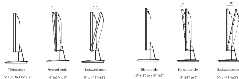
DHI-LM24-L200N
