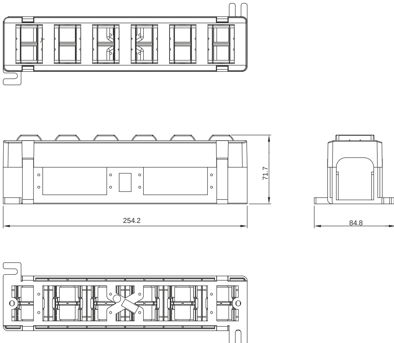
Габаритный чертеж
