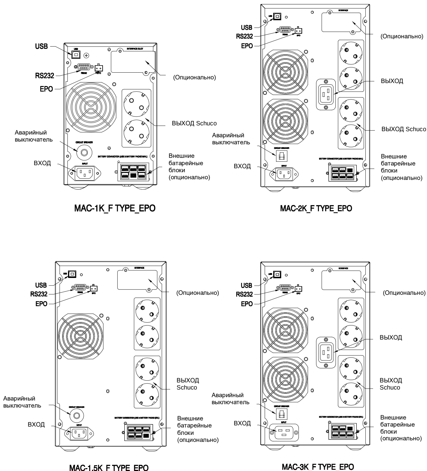
Рис. 4. Задняя панель серии MAC
