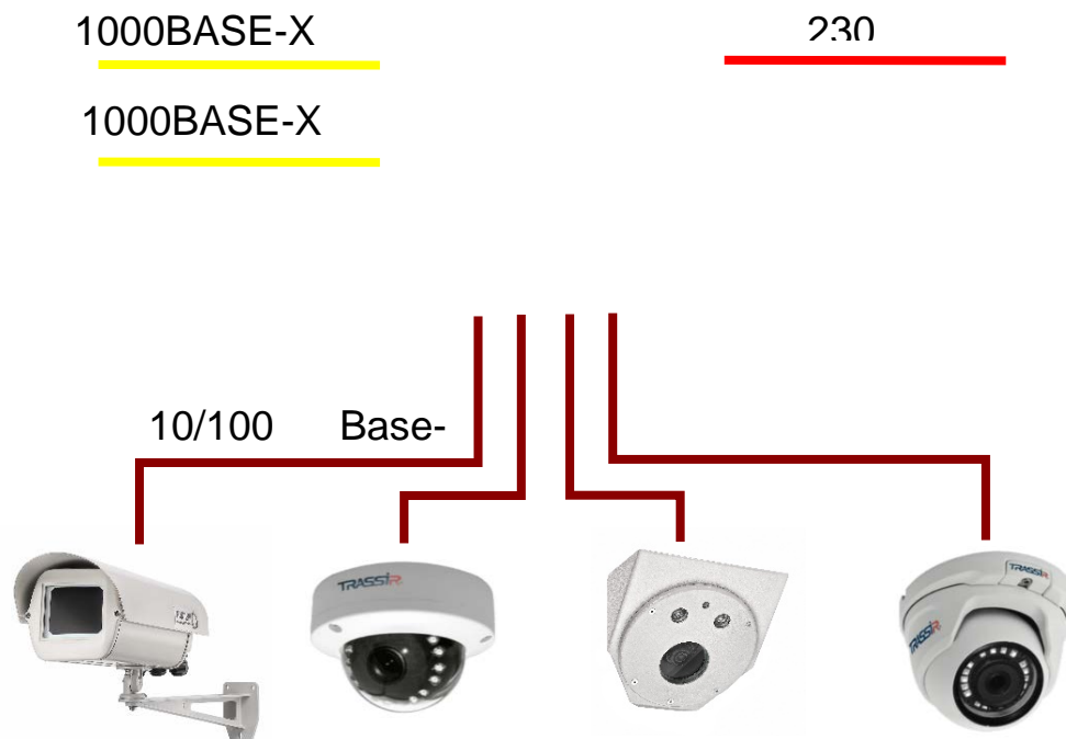
Рисунок 2. Типовая схема подключения коммутатора по двум оптическим кабелям.
