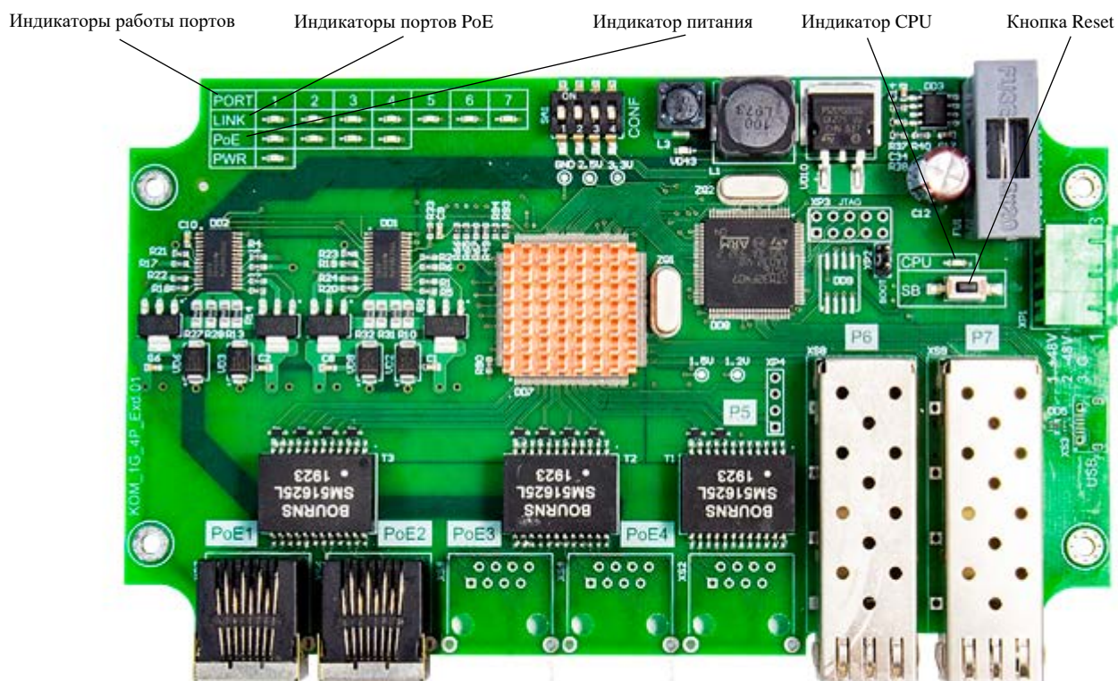
Рисунок 6. Расположение элементов
