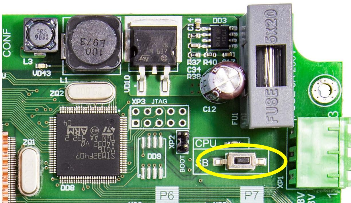
Рисунок 12. Кнопка сброса настроек коммутатора на заводские установки
