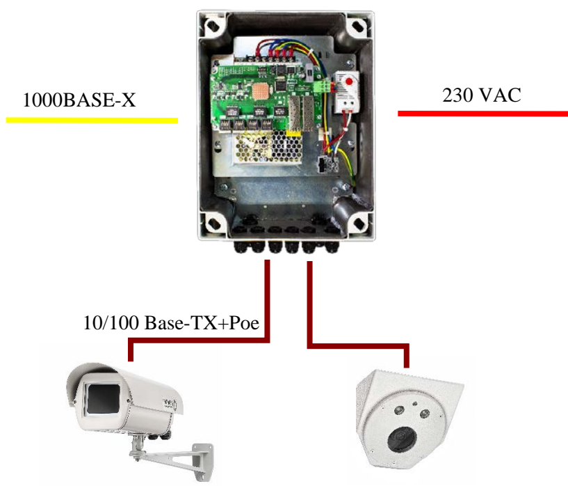
Рисунок 1. Типовая схема подключения коммутатора: по одному оптическому кабелю.
