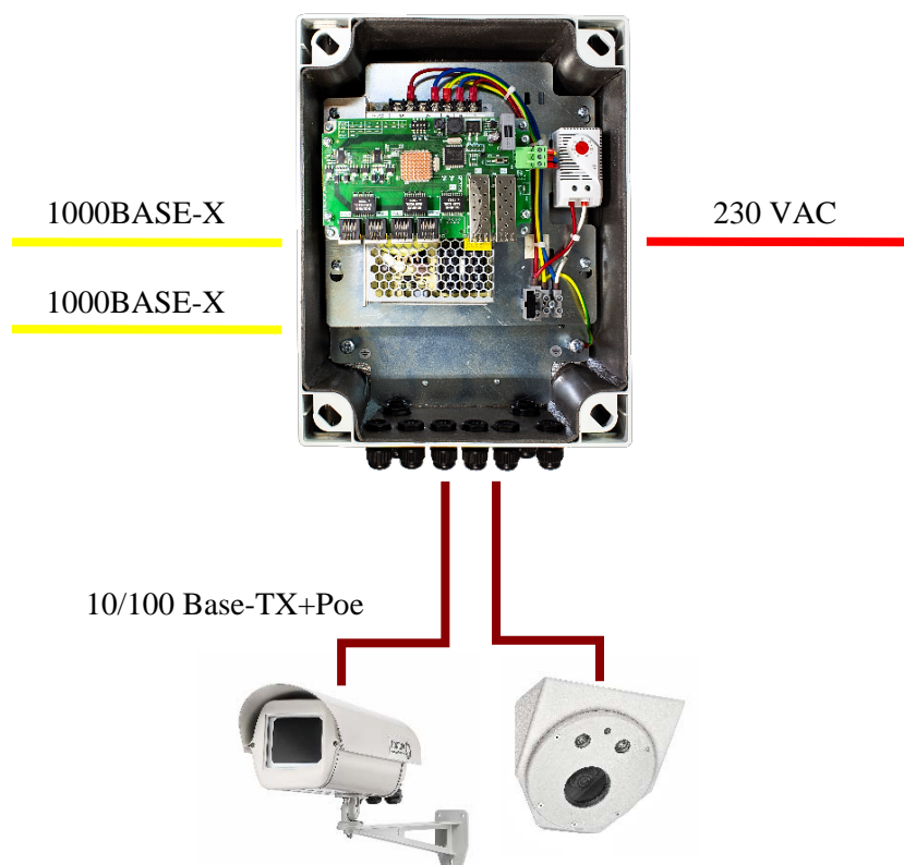
Рисунок 3. Типовые схемы подключения коммутаторов: по двум оптическим кабелям.
