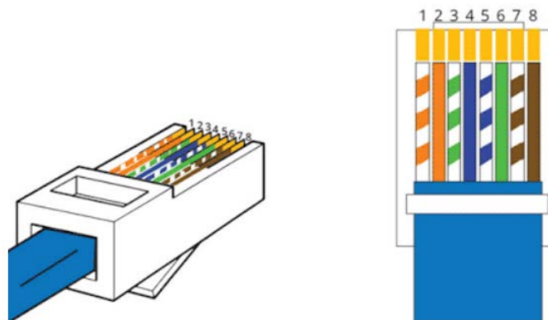
Рисунок 14. Разделка кабеля витая пара
