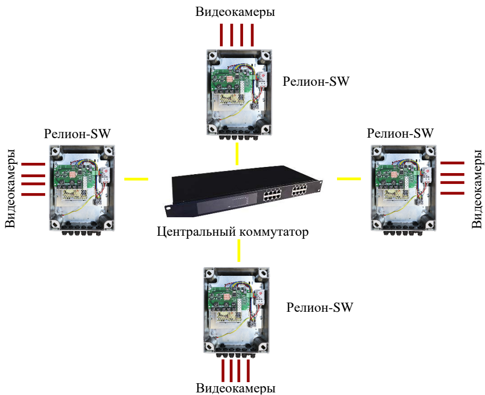
Рисунок 8. Подключение коммутаторов в топологию «звезда»
