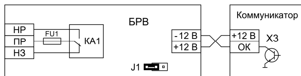
Рис.8 Схема подключения БРВ к универсальному коммуникатору ПКП «Гранит-2...12А»
