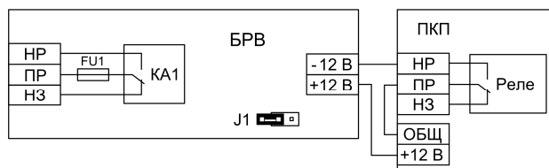
Рис.6 Схема подключения БРВ к штатному реле ПКП
