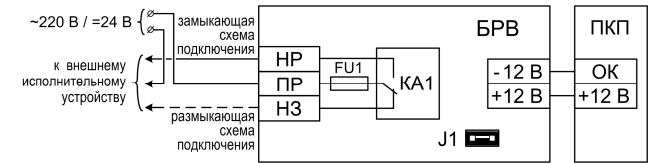
Рис.2 Схема подключения БРВ к выходу ОК ПКП, цепь контроля СЛ подключена
