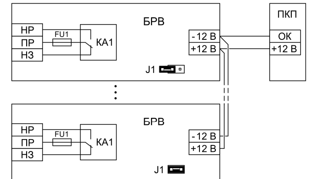
Рис.5 Схема подключения нескольких БРВ к выходу ОК ПКП, контроль СЛ до последнего БРВ
