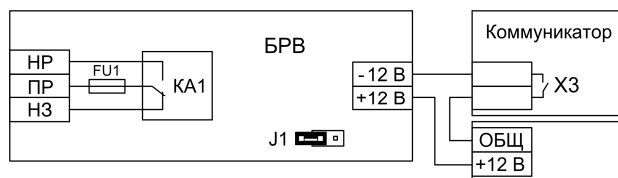
Рис.7 Схема подключения БРВ к GSM коммуникатору ПКП «Гранит-2...12А GSM»
