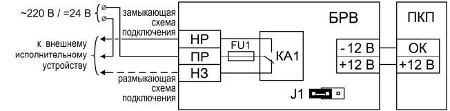
Рис.3 Схема подключения БРВ к выходу ОК ПКП, цепь контроля СЛ отключена
