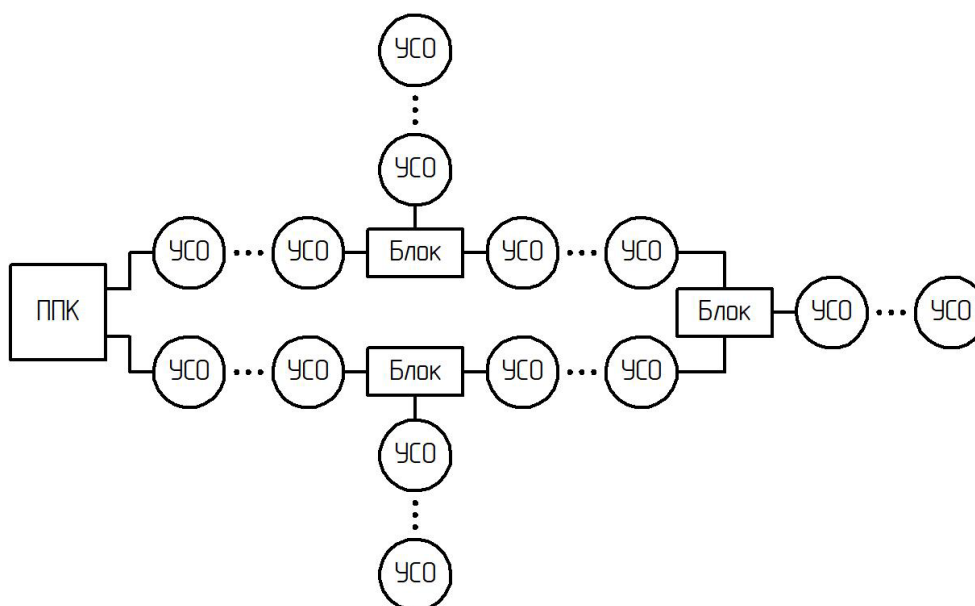
Рисунок 5 – Топология «Смешанная»
