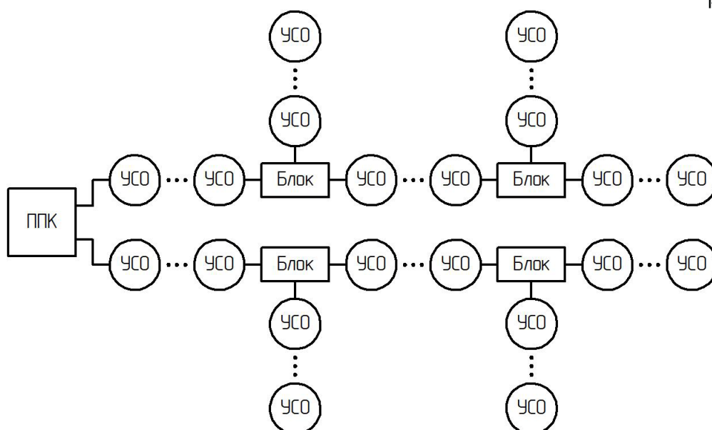
Рисунок 4 – Топология «Дерево»
