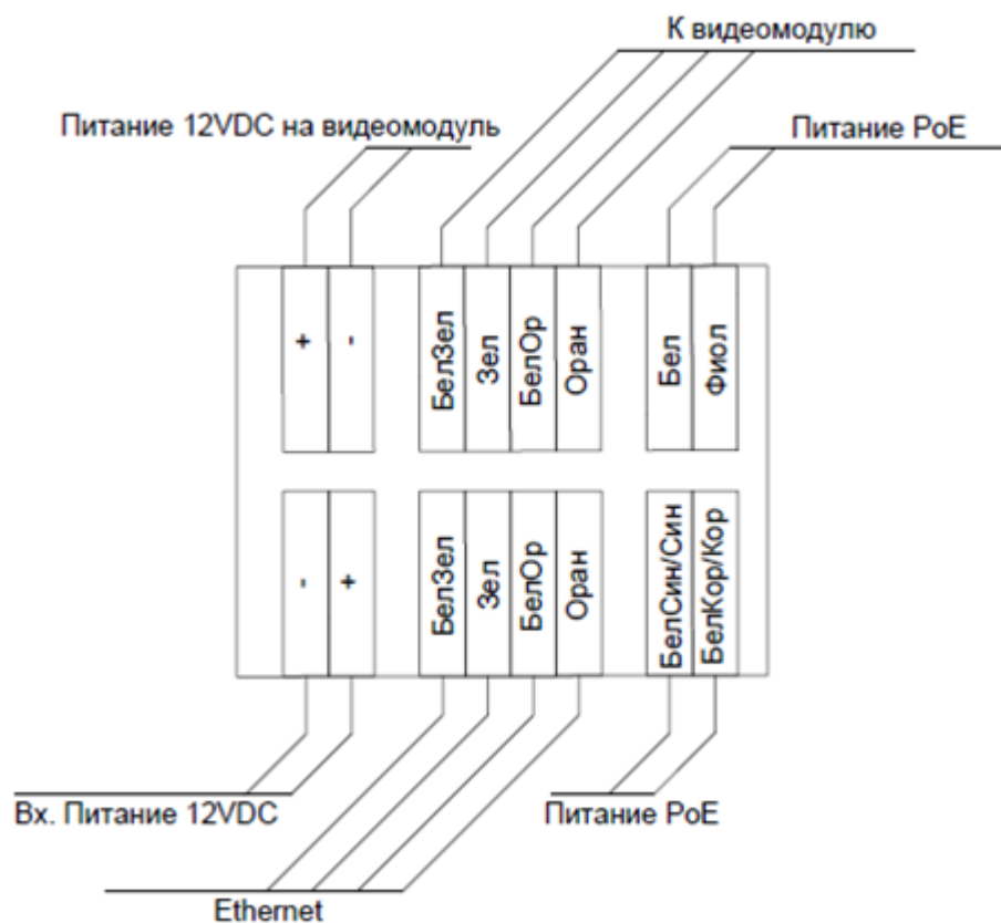
Рисунок 7.6. Схема подключений исполнений IP видеокамер без подогрева
