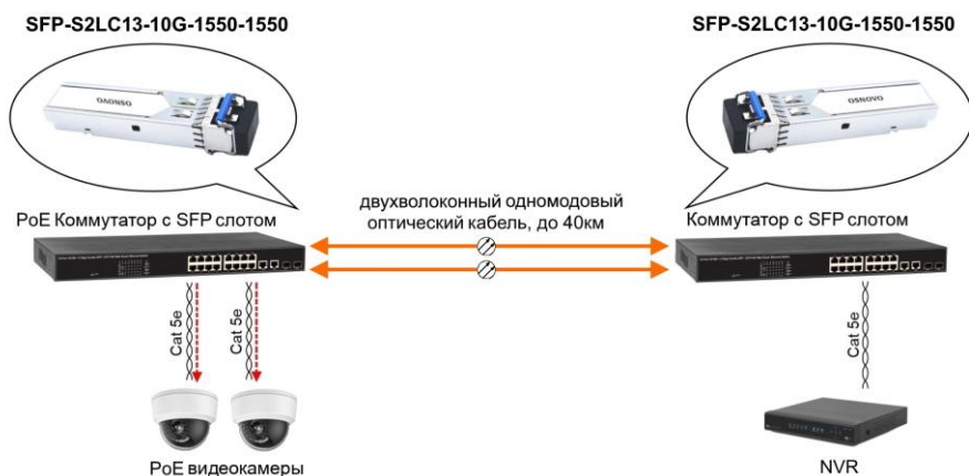
Рис.4 Типовая схема подключения модуля SFP-S2LC13-10G-1550-1550
