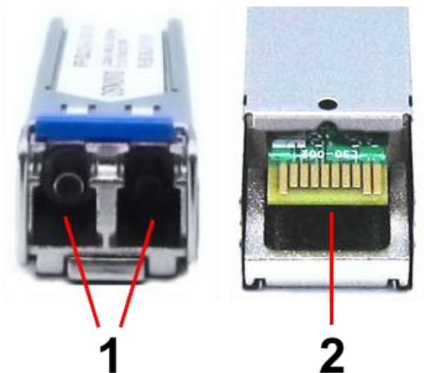
Рис.2 SFP модуль SFP-S2LC13-10G-1550-1550, разъемы спереди/сзади
