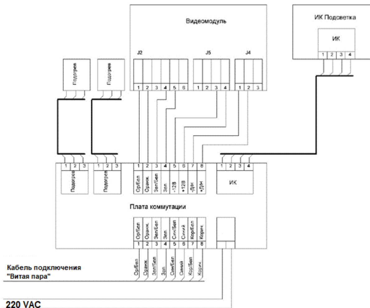
Рисунок 5.6. Коммутационная плата видеокамер исп. «Релион-Ехd-(А/Н)-150(-П)-IP-...» (с питанием 220VAC и обогревом).
