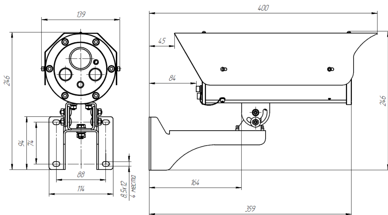
Рисунок А1 – Габаритные размеры с крепежно-юстировочным устройством и чертеж безопасности на Релион-Exd-A-150
