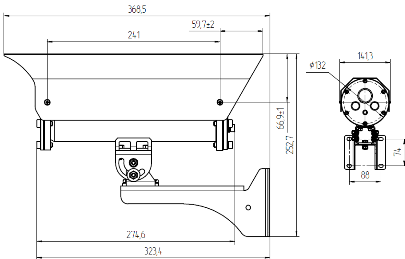
Рисунок А2 – Габаритные размеры с крепежно-юстировочным устройством и чертеж безопасности на Релион-Exd-M/H-150
