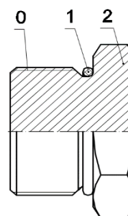
ЗАГЛУШКА – для глушения свободных отверстий под КВ
