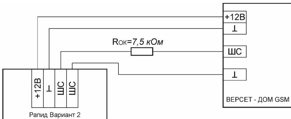
Рис.10. Схема подключения извещателя «Рapid» вариант 2 - датчик движения – к охрannому ШС.
