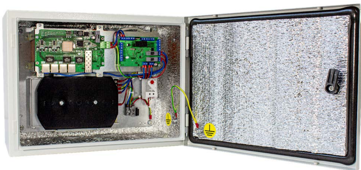
Рисунок 4. Вид изнутри
