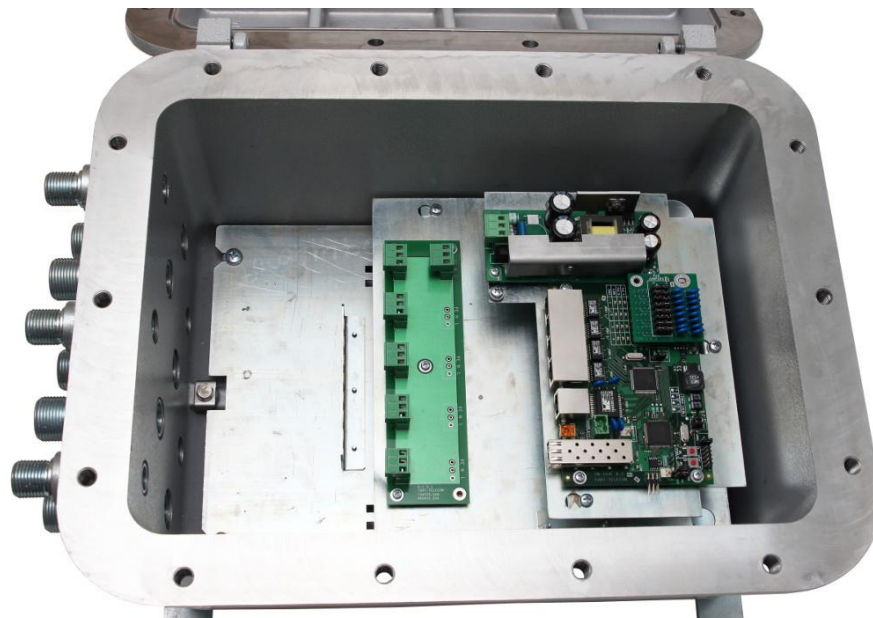
Рисунок 2.6.1 - Плата коммутатора
