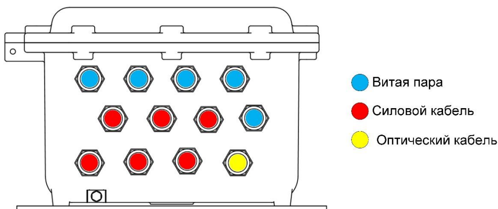
Рисунок 2.3 - Назначение кабельных вводов
