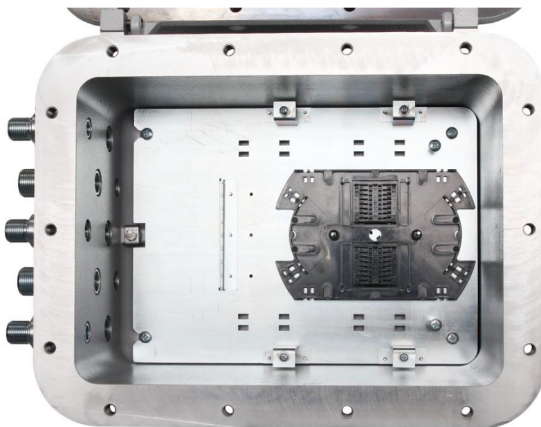
Рисунок 2.4 - Оптический кросс
