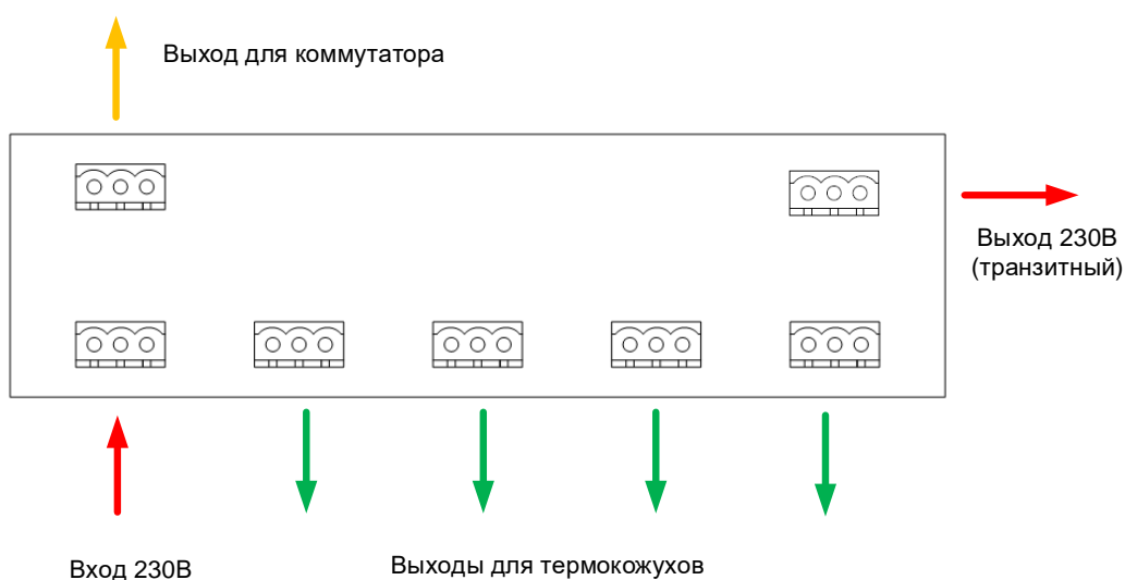
Рисунок 2.5.2 - Назначение разъемов
