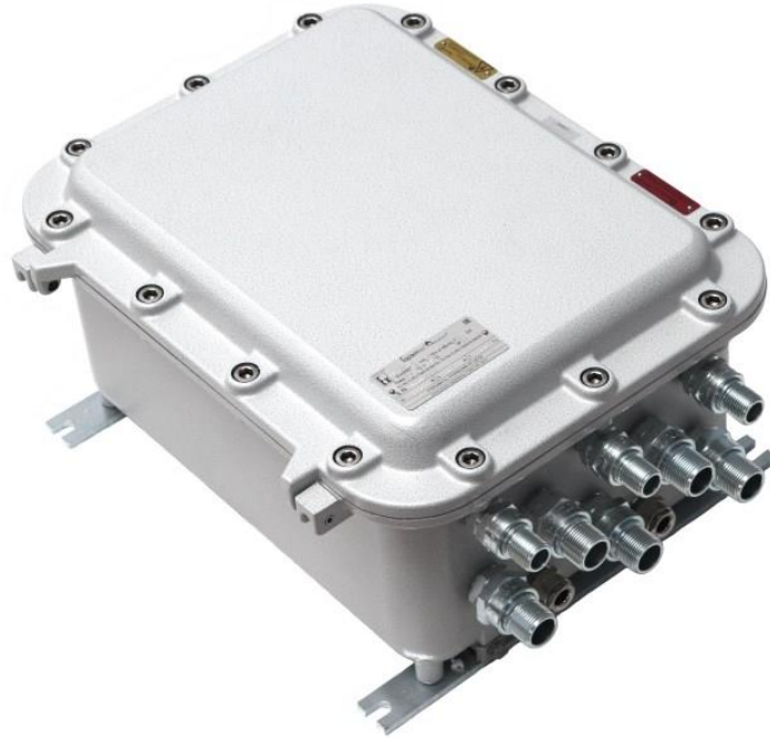
Рисунок 2.1.1 - PSW-1G4F-Ex - вид снаружи
