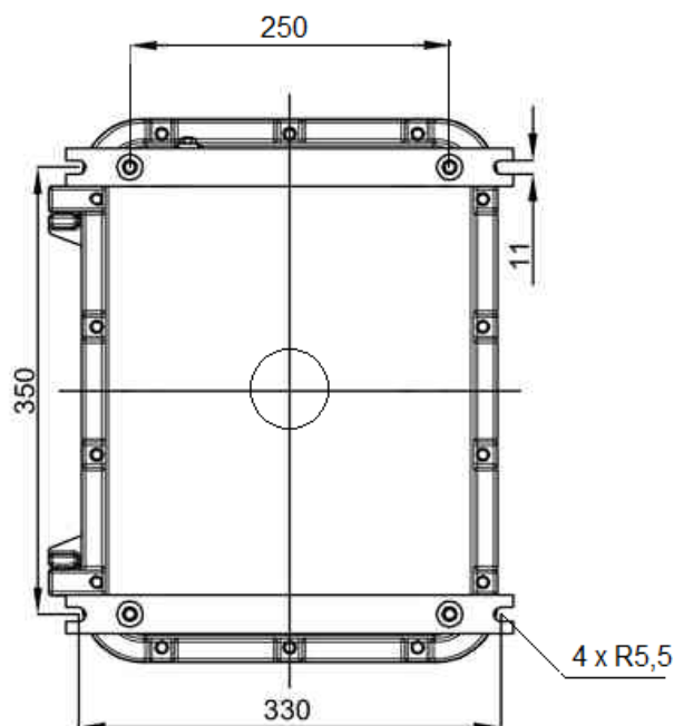
Рисунок 6.1 - Разметка крепления
