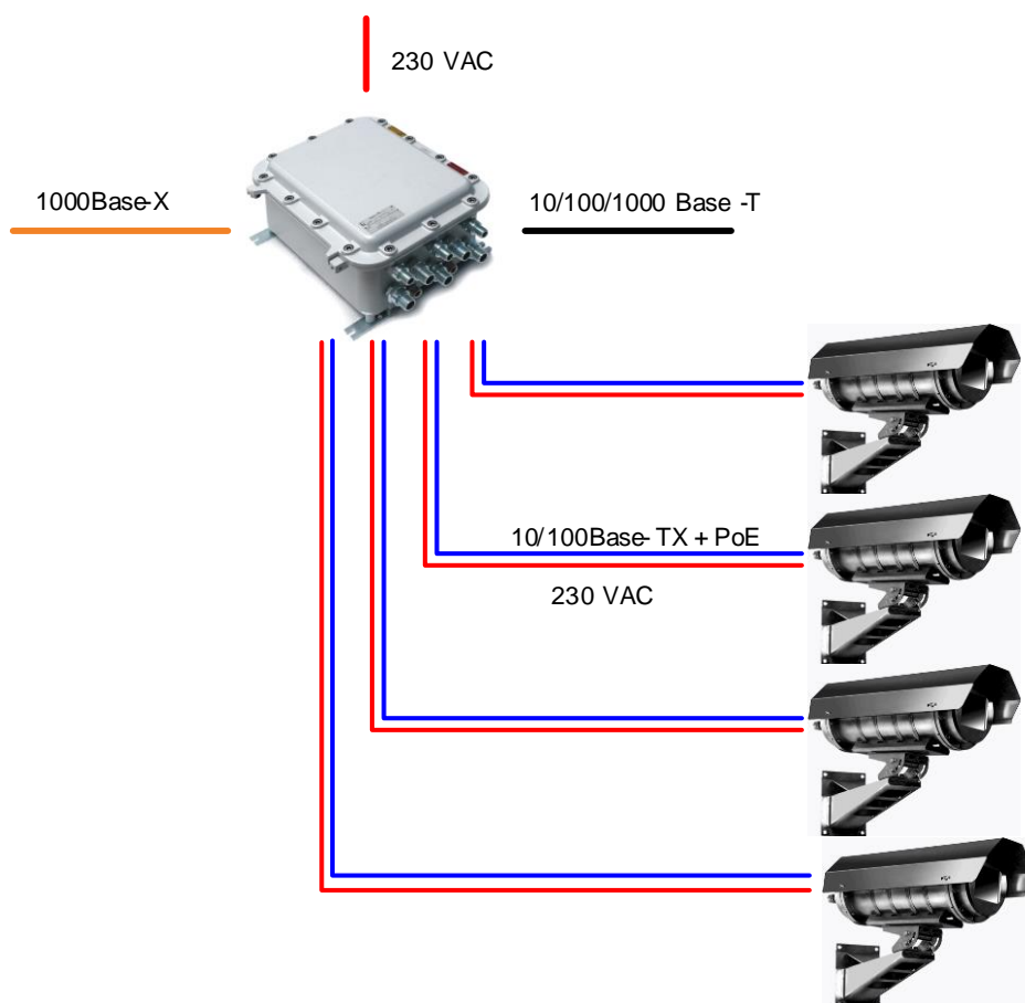
Рисунок 1 - Схема подключения PSW-1G4F-Ex
