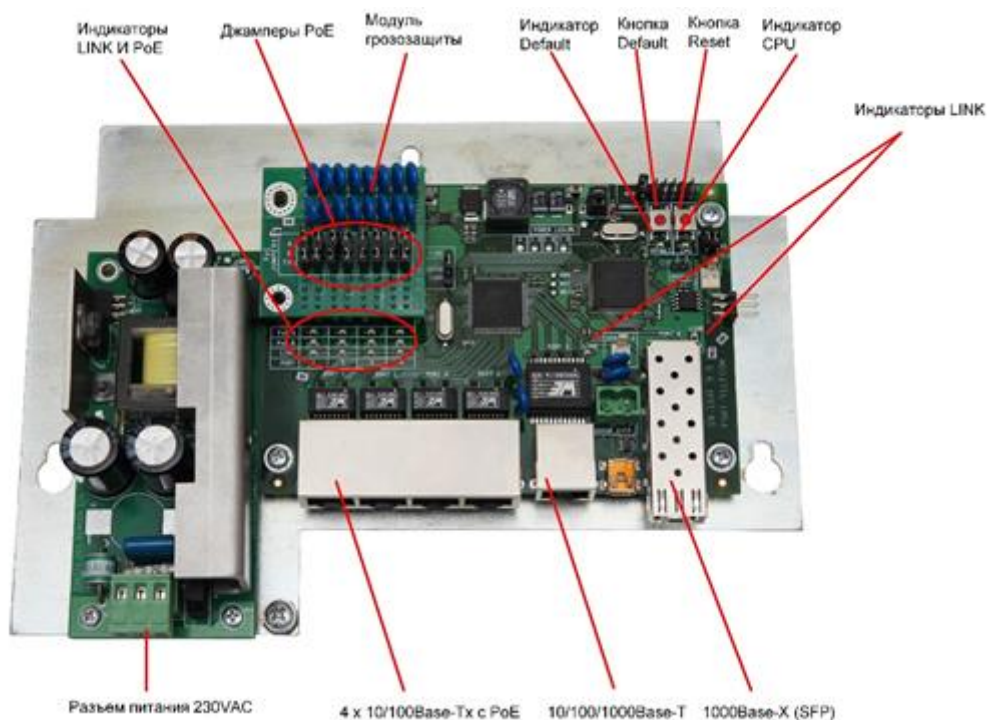
Рисунок 2.6.2 - Расположение элементов на плате коммутатора
