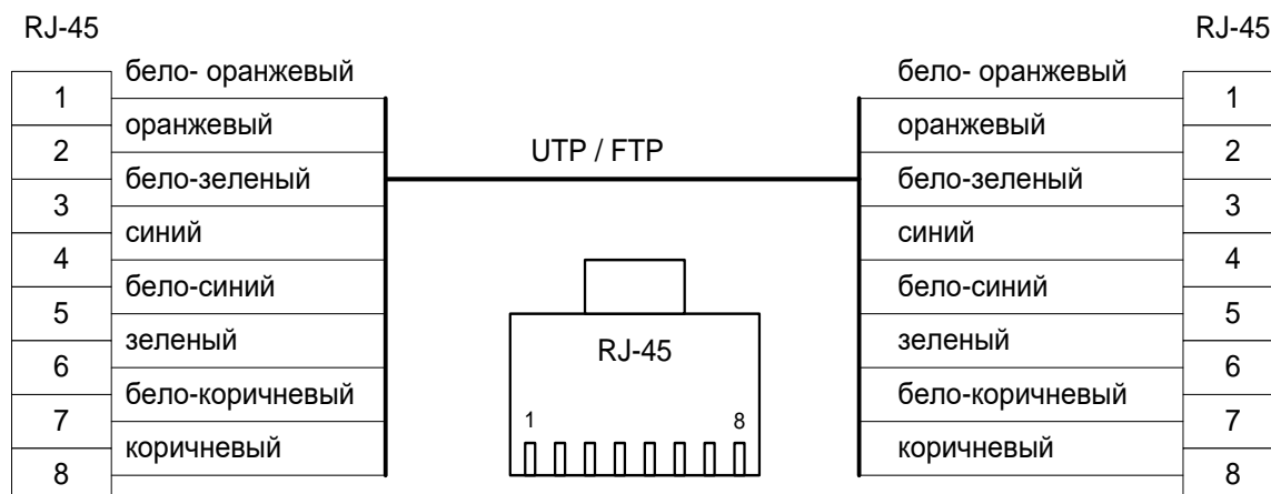
Рисунок 6.4 - Разделка Ethernet кабеля.
