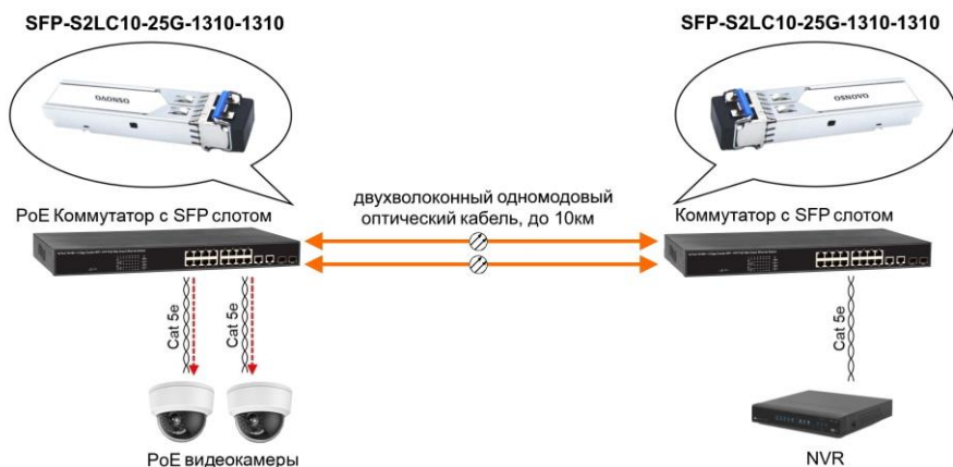
Рис.4 Типовая схема подключения модуля SFP-S2LC10-25G-1310-1310
