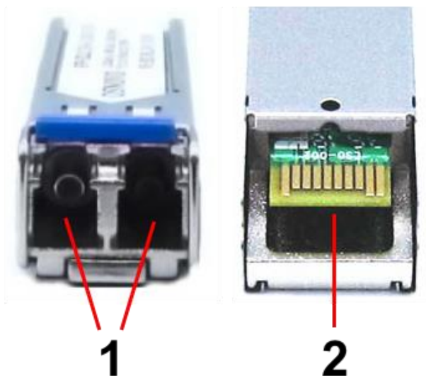
Рис. 2 SFP модуль SFP-S2LC10-25G-1310-1310, разъемы спереди/сзади
