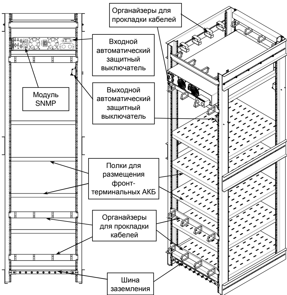
Рисунок 2 — Общий вид изделия сзади, без облочки.
