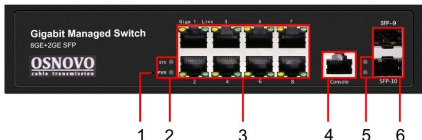
Рис.4 Коммутатор SW-70802/L2, разъемы и индикаторы передней панели
