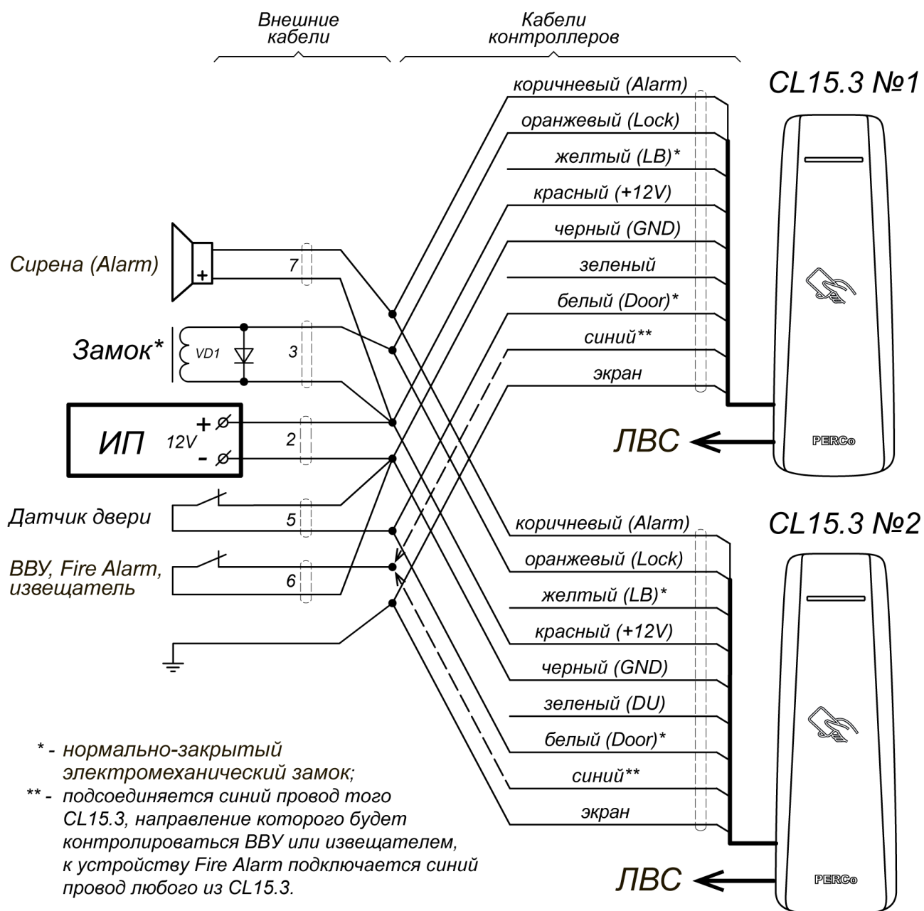
Рисунок 5. Схема параллельного подключения двух контроллеров для управления двусторонней дверью, оборудованной нормально закрытым электромеханическим замком
