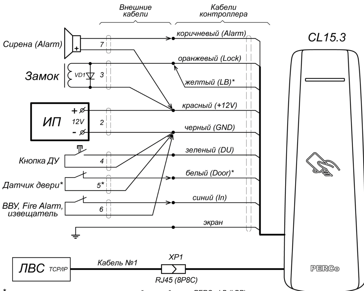
Рисунок 3. Схема подключений контроллера для управления односторонним замком
