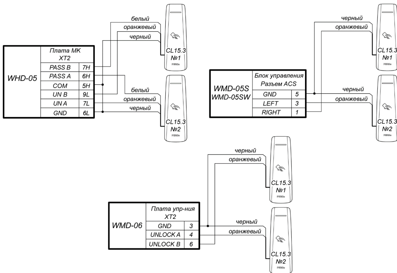
Рисунок 8. Схемы подключений калиток
