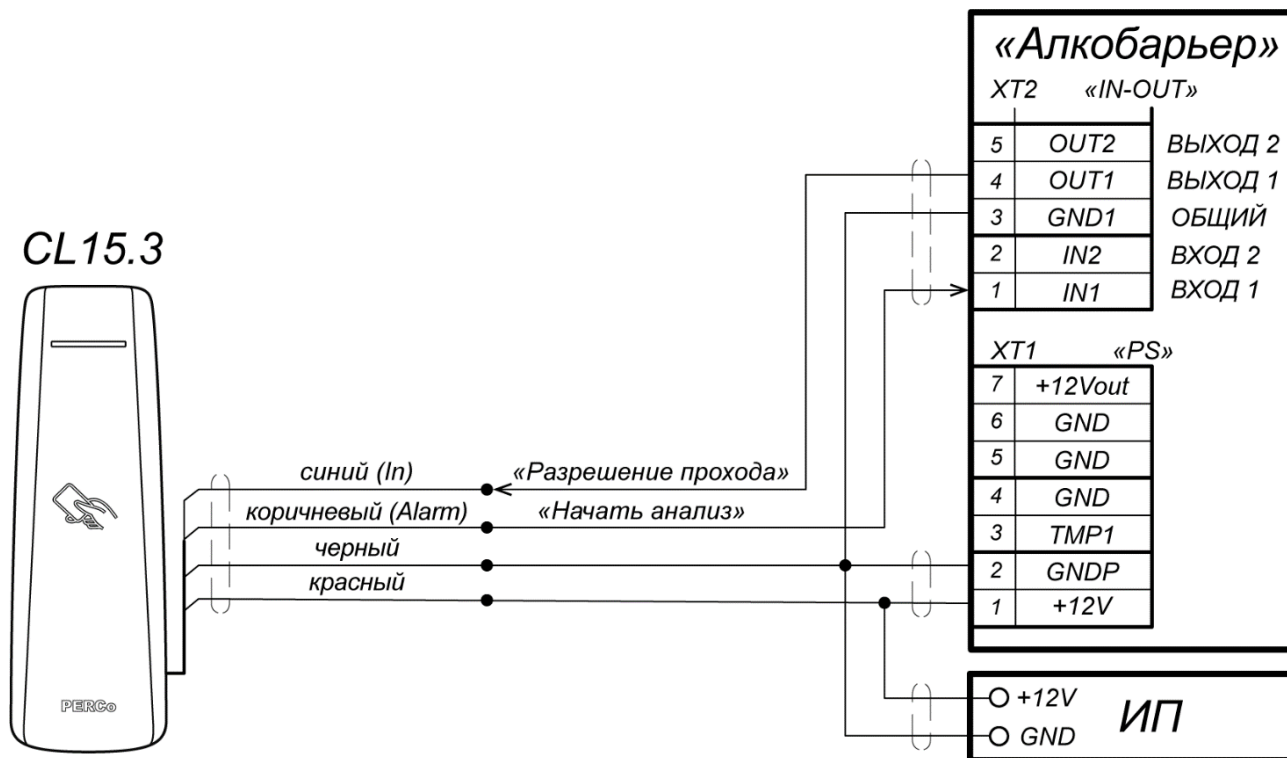
Рисунок 10. Схема подключения ВВУ на примере алкотестера
