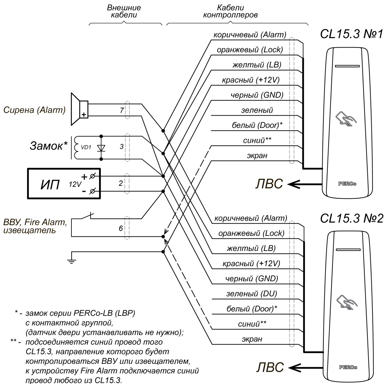
Рисунок 4. Схема параллельного подключения двух контроллеров для управления двусторонней дверью, оборудованной замком с контактной группой типа PERCo-LB (LBP) 1
