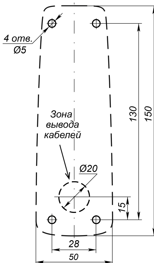
Рисунок 2. Разметка отверстий для установки контроллера (пунктиром показаны габариты корпуса контроллера)
