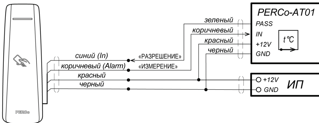
Рисунок 13. Схема подключения пирометра PERCo-AT01 к контроллеру CL15.3
