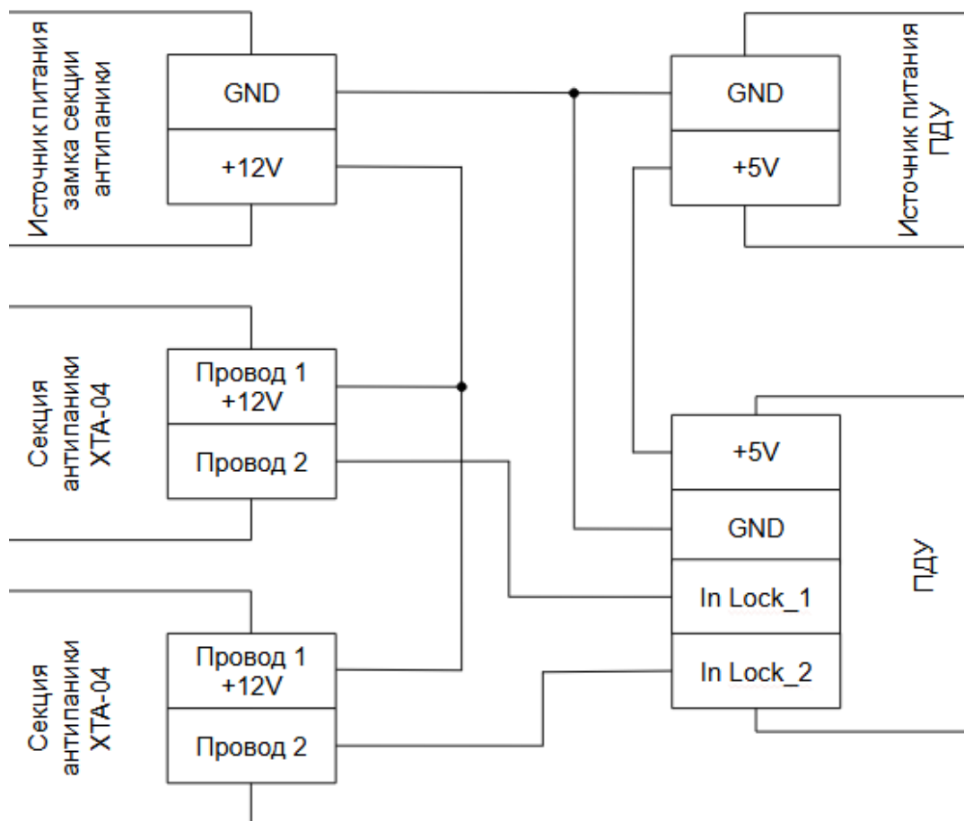
Рисунок 8.3 Схема подключения секции Антипаники «ХТА-04» к ПДУ «AG-02», «TG-04», «TC-06»
