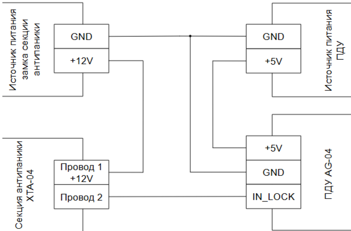
Рисунок 8.2 Схема подключения секции Антипаника «ХТА-04» к ПДУ «AG-04»
