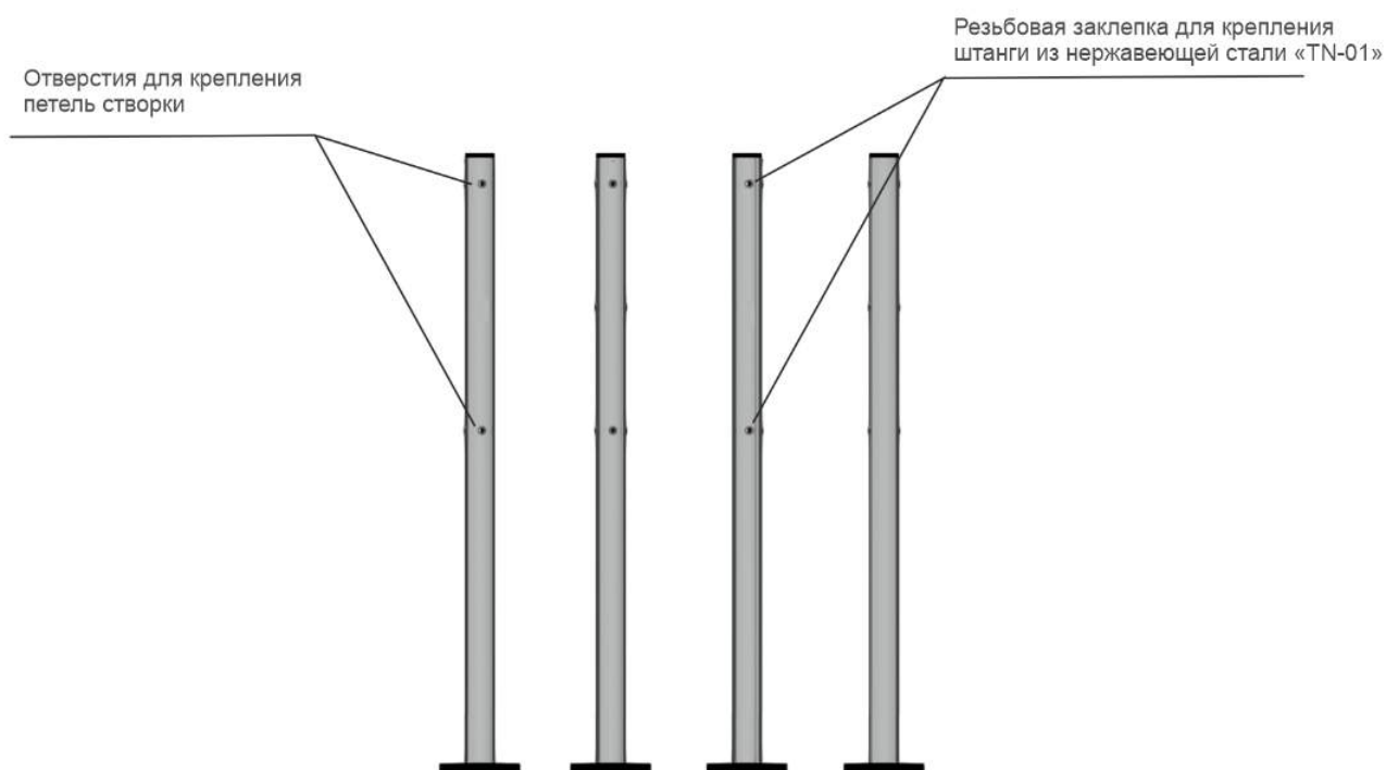
Рисунок 6.1.2 Стойка петельная «ХТА-04»
