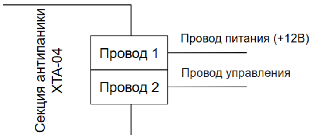
Рисунок 8.1 Назначение проводов секции Антипаника «ХТА-04»
