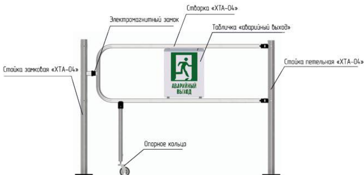
Рисунок 6.1 Состав секции Антипаника с электромагнитным замком «ХТА-04»
