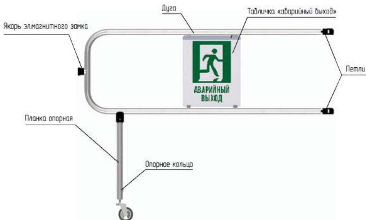
Рисунок 6.2.1 Створка «ХТА-04»
