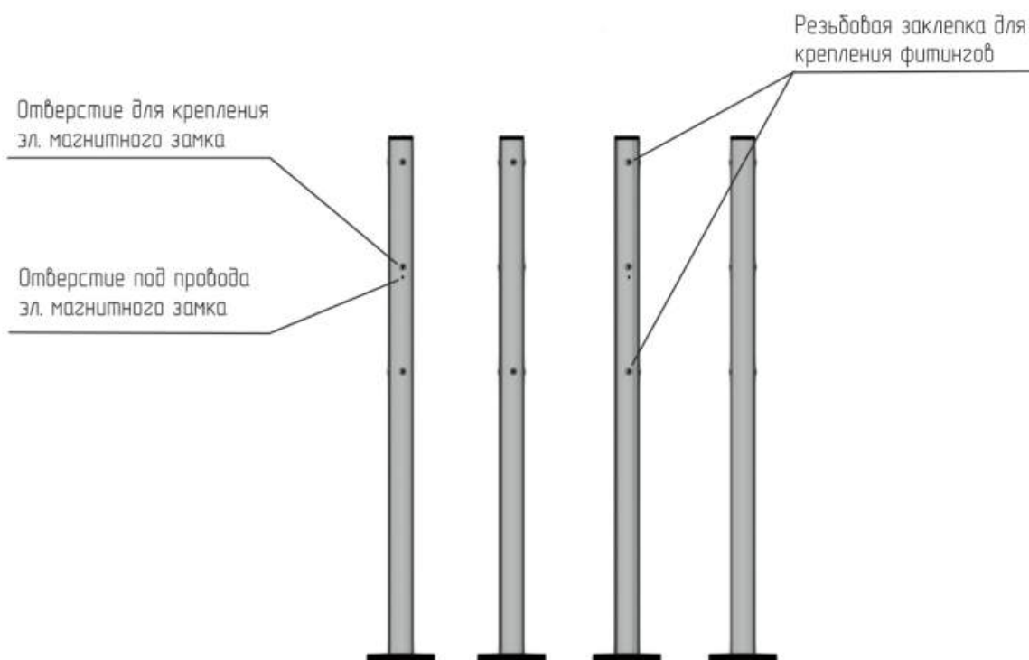
Рисунок 6.1.1 Замковая стойка «ХТА-04»
