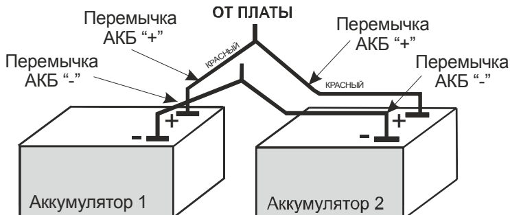
Рисунок 4. Параллельное подключение двух аккумуляторов.
