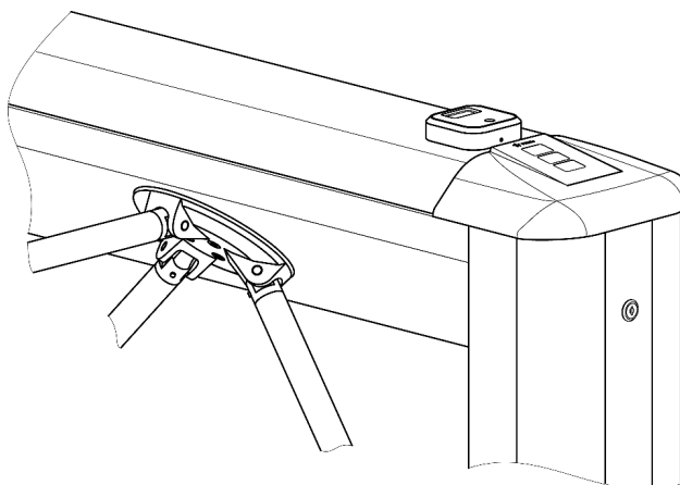
Рисунок 31. Место установки пирометра PERCo-AT01 на крышку ЭП
