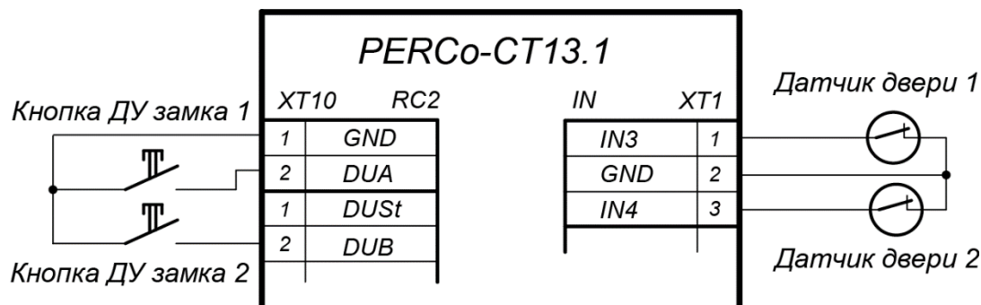
Рисунок 15. Схема подключений кнопок ДУ и датчиков двери
