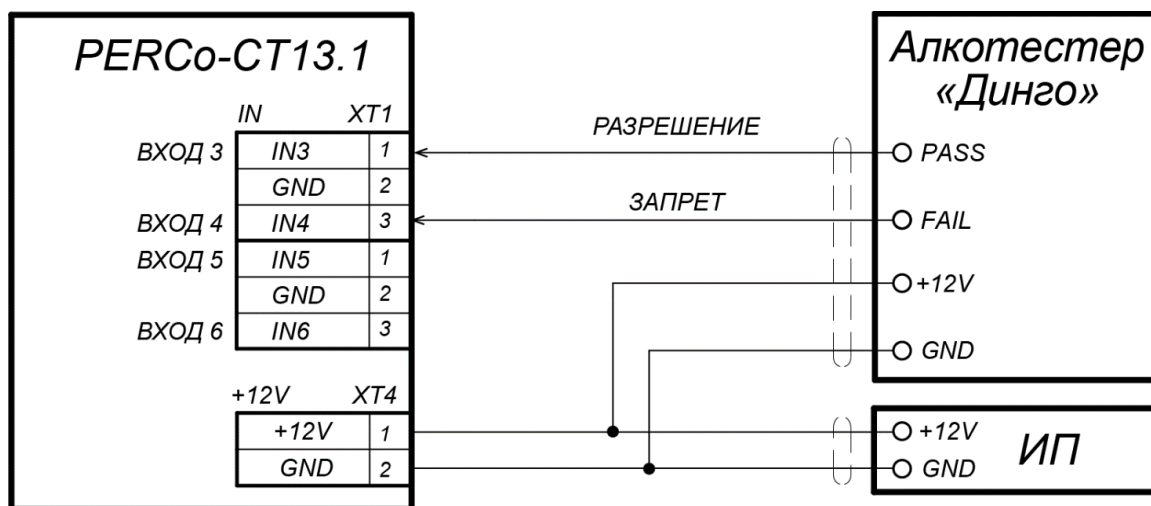
Рисунок 28. Схема подключения алкотестера «Динго В-02» (ООО СИМС-2)
