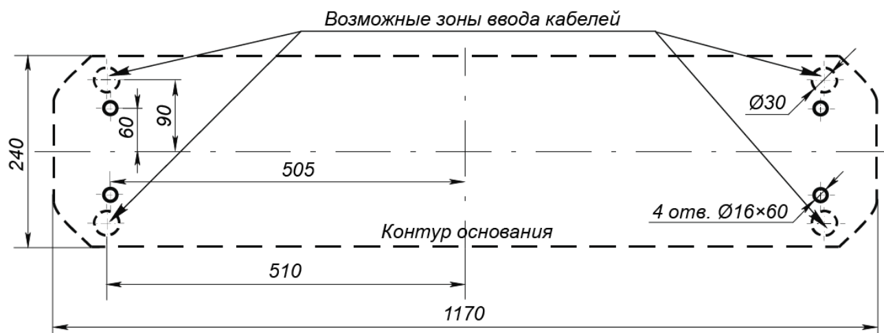
Рисунок 11. Схема разметки для установки стойки ЭП 1
