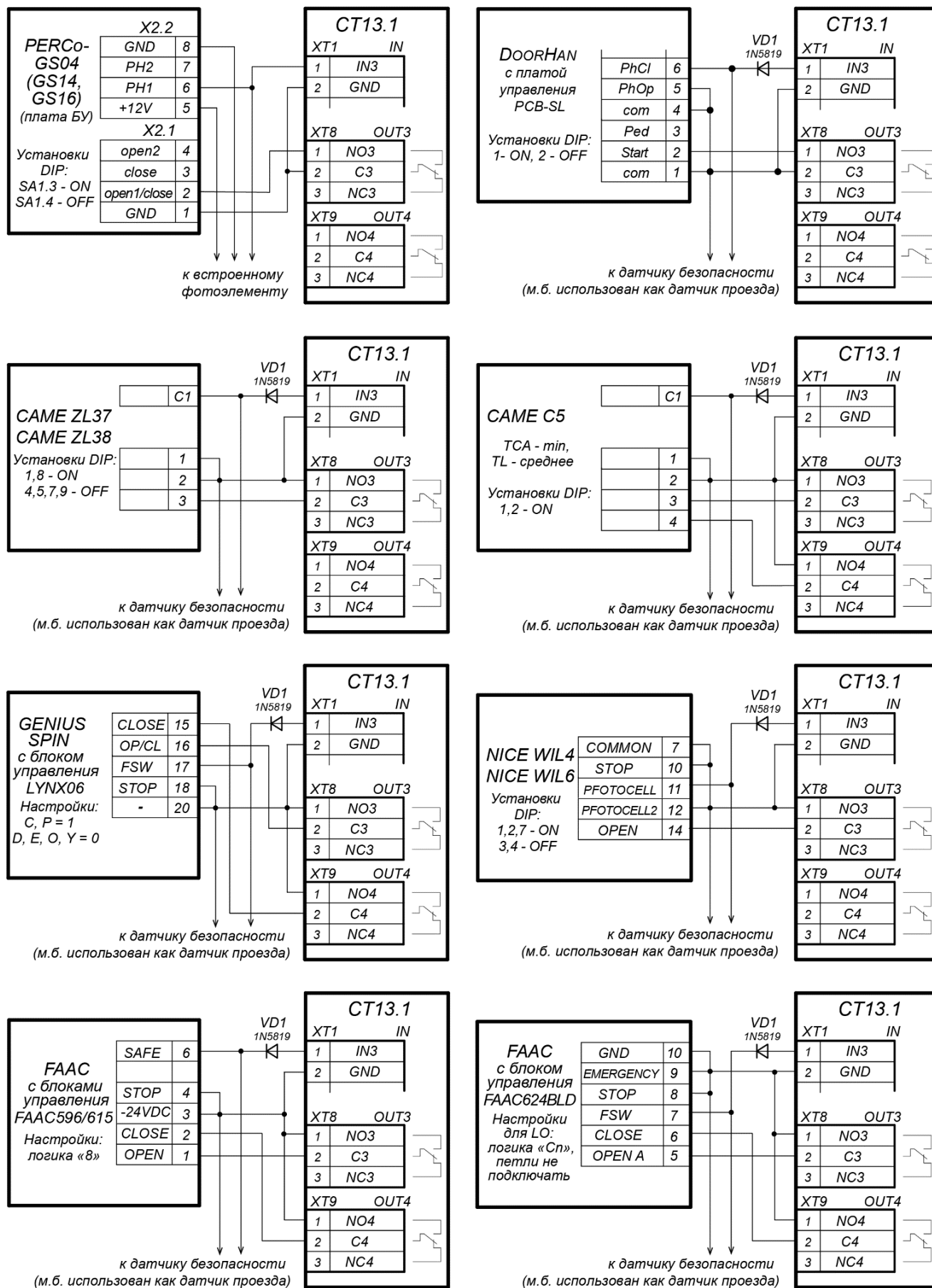
Рисунок 18. Примеры схем подключения шлагбаумов к контроллеру АТП
