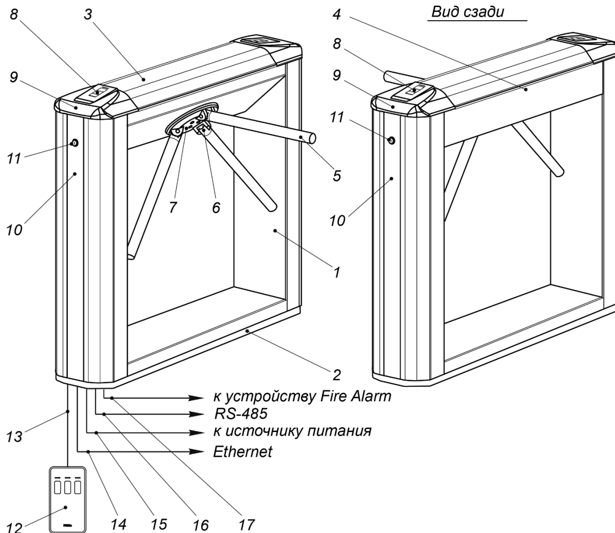
Рисунок 2. Устройство ЭП
