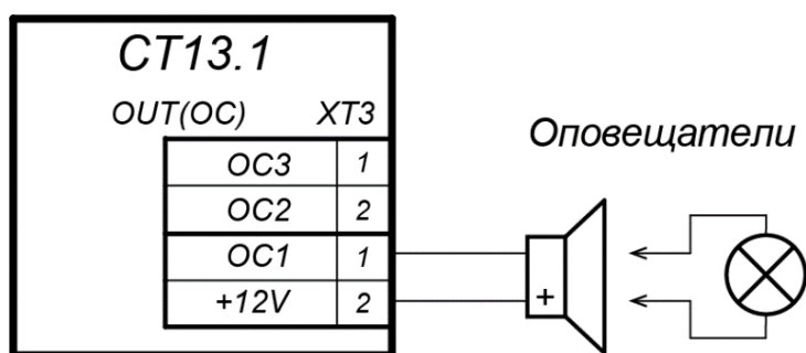
Рисунок 21. Схема подключений дополнительного оборудования к выходам контроллера типа «Открытый коллектор»
