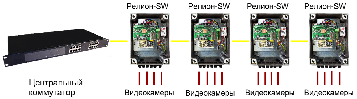
Рисунок 9. Подключение коммутаторов в топологию «линия»
