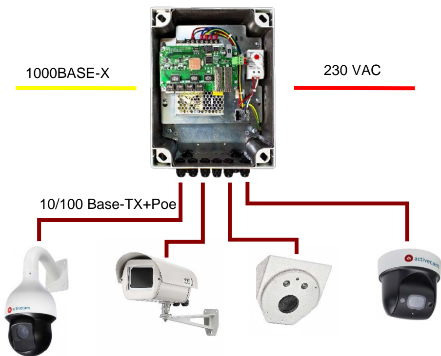
Рисунок 1. Типовая схема подключения коммутаторов по одному оптическому кабелю.
