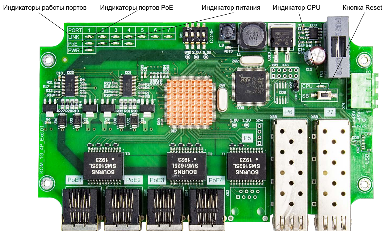
Рис. 6. Расположение элементов
