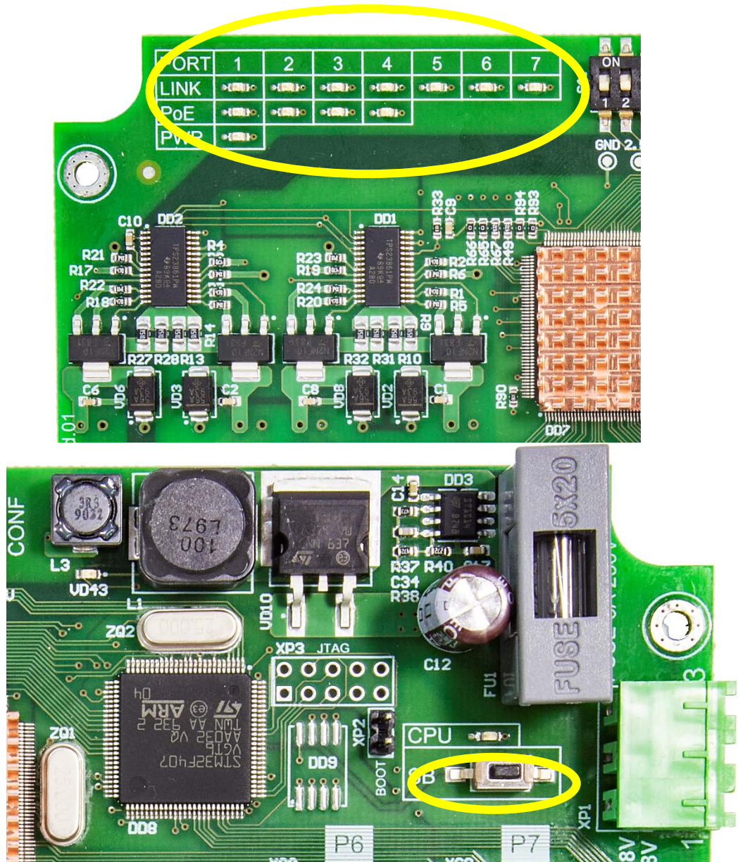
Рисунок 11. Расположение элементов индикации и настройки на плате коммутатора
