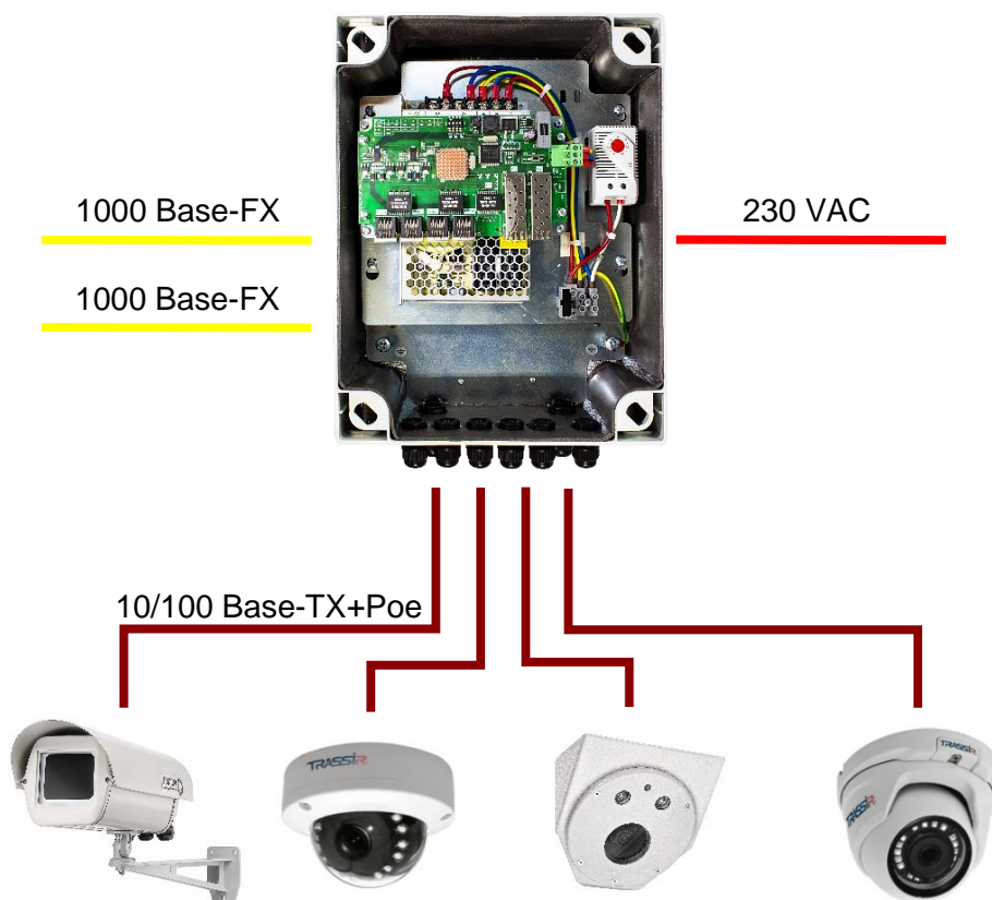
Рисунок 3. Типовые схемы подключения коммутаторов: Релион-SW-2G-4Poe+/60W; Релион-SW-2G-4Poe+/150W; Релион-SW-2G-4Poe+/240W по двум оптическим кабелям.
