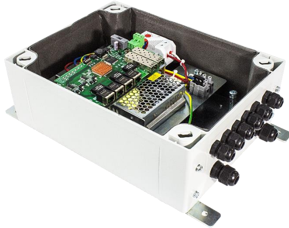
Рисунок 5. Релион-SW-2G-4Poe+/60W вид изнутри
