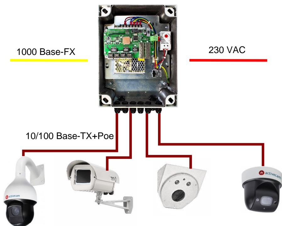
Рисунок 1. Типовая схема подключения коммутаторов: Релион-SW-2G-4Poe+/60W; Релион-SW-2G-4Poe+/150W; Релион-SW-2G-4Poe+/240W по одному оптическому кабелю.
