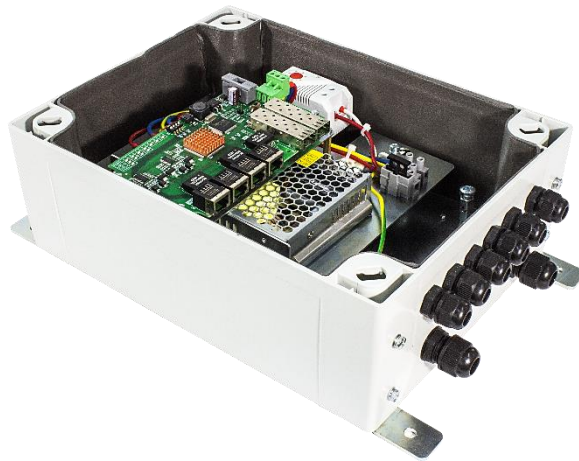
Рисунок 6. Релион-SW-2G-4Poe+/150W вид изнутри
