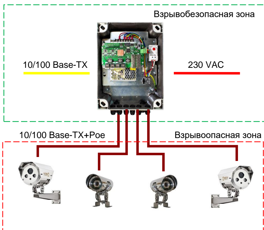
Рисунок 2. Типовая схема подключения коммутаторов: Релион-SW-2G-4Poe+/60W; Релион-SW-2G-4Poe+/150W; Релион-SW-2G-4Poe+/240W по одному оптическому кабелю.
