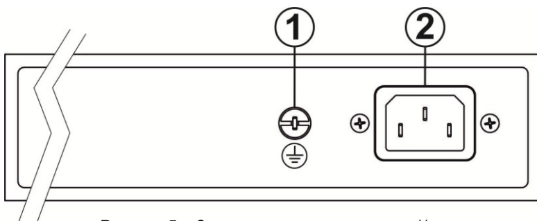
Рисунок 5 – Задняя панель коммутатора**
