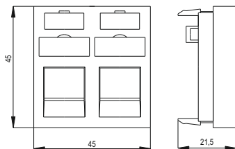
Рисунок 10 – Вставка CS6-22M / Figure 10 – CS6-22M insert
